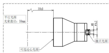
NTD29IR055W223M42-I
